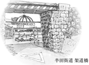
半田街道 架道橋
