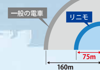
一般の電車では半径160mは必要です。
